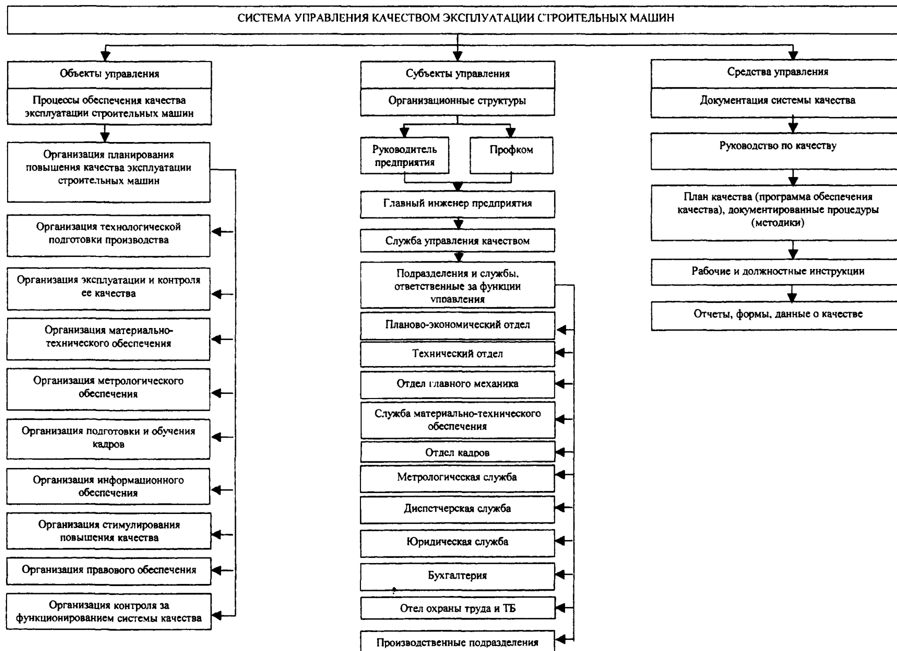
Рис.1. Схема системы управления качеством эксплуатации строительных машин
