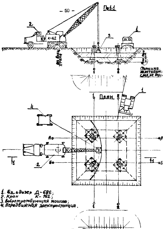
Рис.10. Схема обратной засыпки котлованов под фундаменты опор У35-2, У110-1, У110-2
