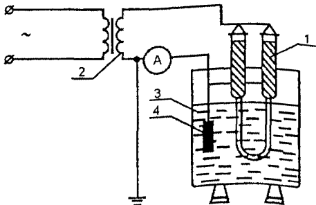
Рис. 2.1. Принципиальная схема испытания электрической прочности изоляции рукоятки и провода указателя на напряжение: 1 – испытываемый указатель; 2 – испытательный трансформатор; 3 – ванна с водой; 4 – электрод
