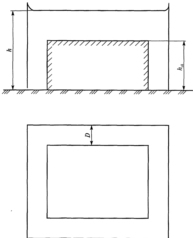
Рис. 3.5. Зона защиты замкнутого тросового молниеотвода
