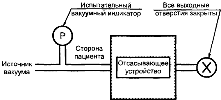
Рисунок А.5 — Схема измерения максимального допустимого вакуума
