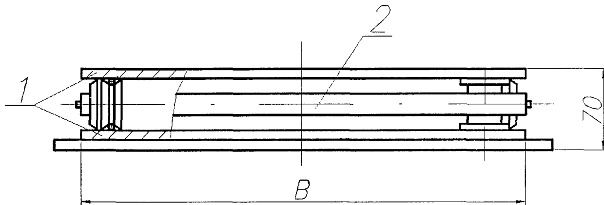
1 – плита опорная; 2 – обойма катковая
