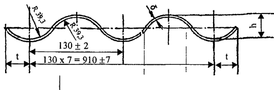
Рис. II.1.1. Профиль гофрированного листа: H=32,5\pm 3 мм; \delta=1,5 ; 2 и 2,5 мм; t=32,5\pm 7,5 мм
