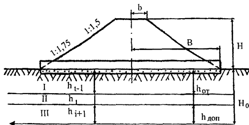
Рис.П.7.1. Схема к расчету осадок труб на оттаивающих грунтах
