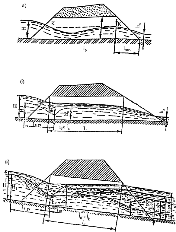
Рис. П.3.1. Схема протекания воды в равнинной трубе при безнапорном режиме: а – «короткая»; б – «длинная»; в – «незатопленная» ( h_{62}, h_{63} ) и «затоплены» с нижнего бьефа ( h_{64} ).
