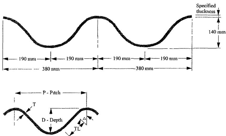
Рис. П.1.4. Профиль гофрированного листа: толщина листа 3,5-7,1 мм; углы изгиба гофра 49,75°-50,43°; прямая вставка 110,78-106,15 мм
