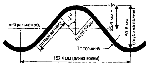
Рис. II.1.2. Профиль гофрированного листа: толщина листа 3,0-7 мм; углы изгиба гофра 44,53^\circ - 46,08^\circ ; прямая вставка 43,24-47,88 мм
