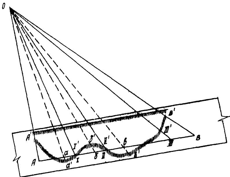
Рис. 9. Пренос отметок с использованием восковок
