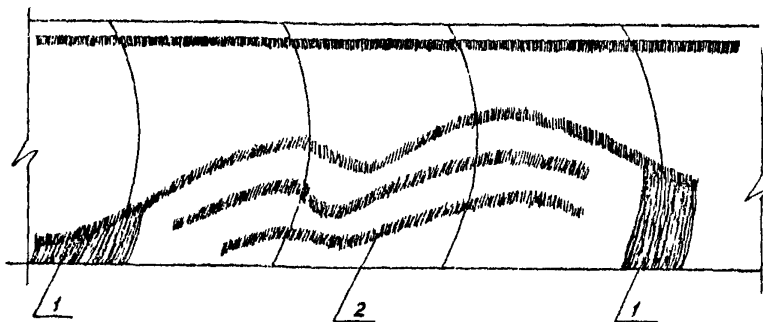
Рис. 5. Изображение песчаных и илистых грунтов на ленте самописца: 1 - ил; 2 - песок
