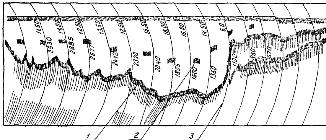
Рис. 4. Лента самописца: 1 - линия записи глубин; 2 - линия записи измерений скорости; 3 - оперативные отметки
