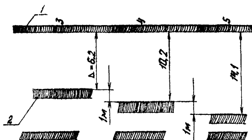
Рис. 2. Батиграмма тарирования: 1—начальная линия; 2—линия записи сигнала, отраженного от диска
