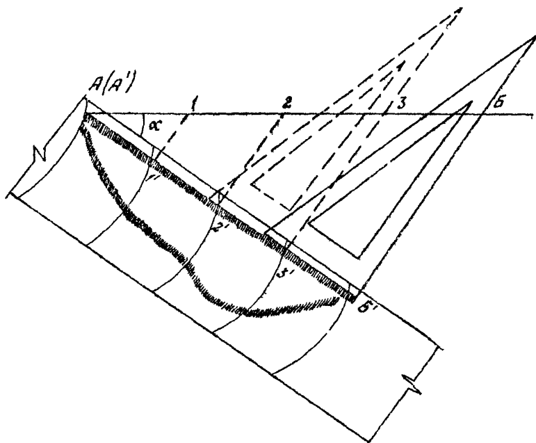
Рис. 8. Перенос отметок на план способом треугольника
