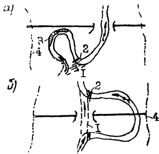
Рис. 12. Схема спрямлений излучин русла: а - спрямляемая излучина, угрожающая пойменной насыпью; б - расположение моста на спрямленном русле: 1 - спрямление; 2 - запруда; 3 - укрепление берега; 4 - граница разлива при УВВ
