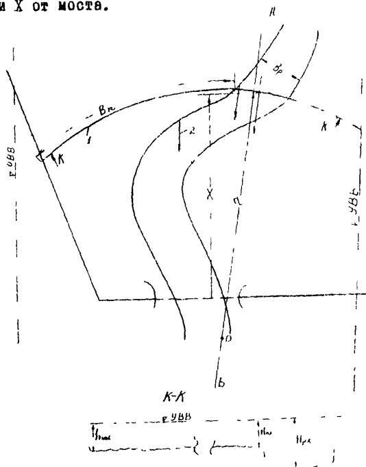
Рис.10. Нанесение пойменного живого сечения на план участка:
