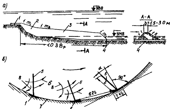
Рис. 14. Схема защиты размываемого берега полузапрудой:
