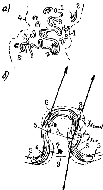
Рис. 1. План свободно меандрирующего русла: а - участок долины; б - характерная излучина; I - излучины русла; 2 - старицы; 3 - прируслов- вые впадины; 4 - границы поймы; 5 - перекаты; 6 - плесовые ложины; 7 - начальное положение вогнутых берегов; 8 - то же после смещения; 9 - направление будущего спрямления центральной излучины
