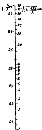
Рис. II. Значение гиперболической функции Sh \frac{4.75h_{max}}{L}
