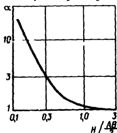
Рис.5. График зависимости (по М.Ф.Монтрею)
