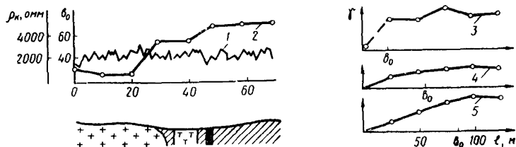
рис.2. Пример применения вариограмм (по Г.А.Соловьеву)
