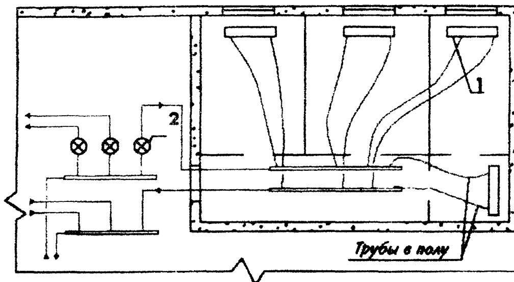
Схема 1. Лучевая схема системы отопления
