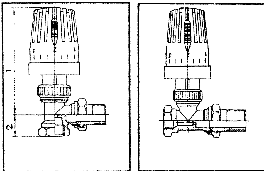
Схема радиаторного термостата
