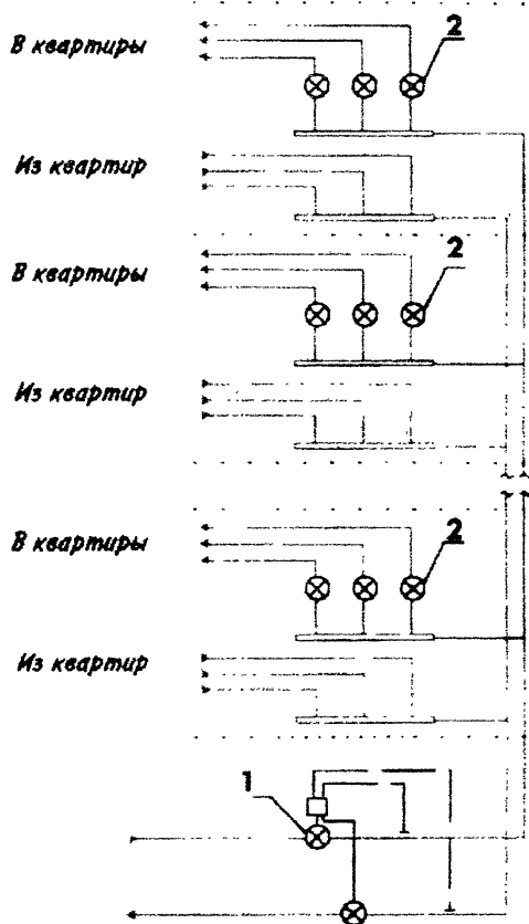
Схема 3. Схема поквартирного учета тепла
