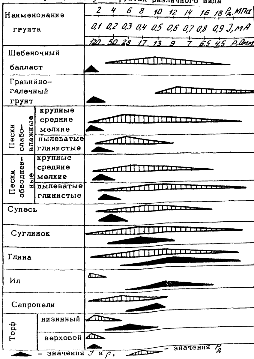
Приложение 5 Диаграмма распределения условного динамического сопротивления R_d , силы тока J и удельного электрического сопротивления \rho в грунтах различного вида
