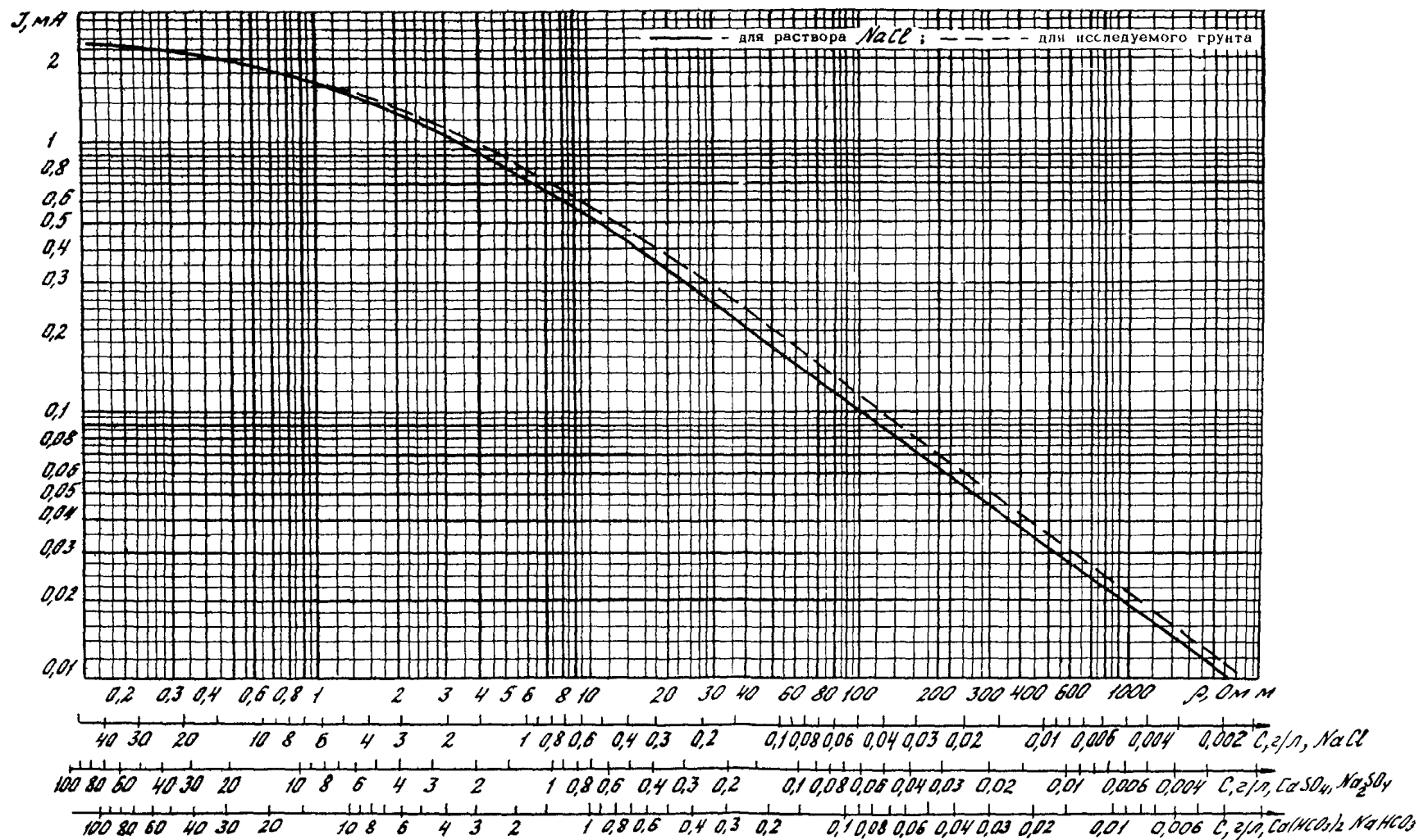
ГРАФИК ИЗМЕНЕНИЯ СИЛЫ ТОКА J В ЗАВИСИМОСТИ ОТ УДЕЛЬНОГО ЭЛЕКТРИЧЕСКОГО СОПРОТИВЛЕНИЯ \rho РАСТВОРА NaCl И ИССЛЕДУЕМЫХ ГРУНТОВ
