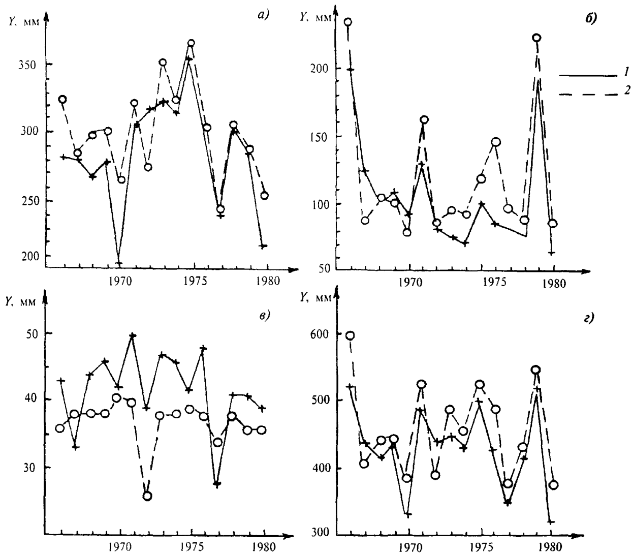
а) — весеннее половодье; б) — летне-осенний сезон; в) — сезон зимней межени; з) — годовое сто Рисунок А.5 — Сравнение фактических (1) и рассчитанных (2) слоев стока р. Вага — с. Усть-Сюма
