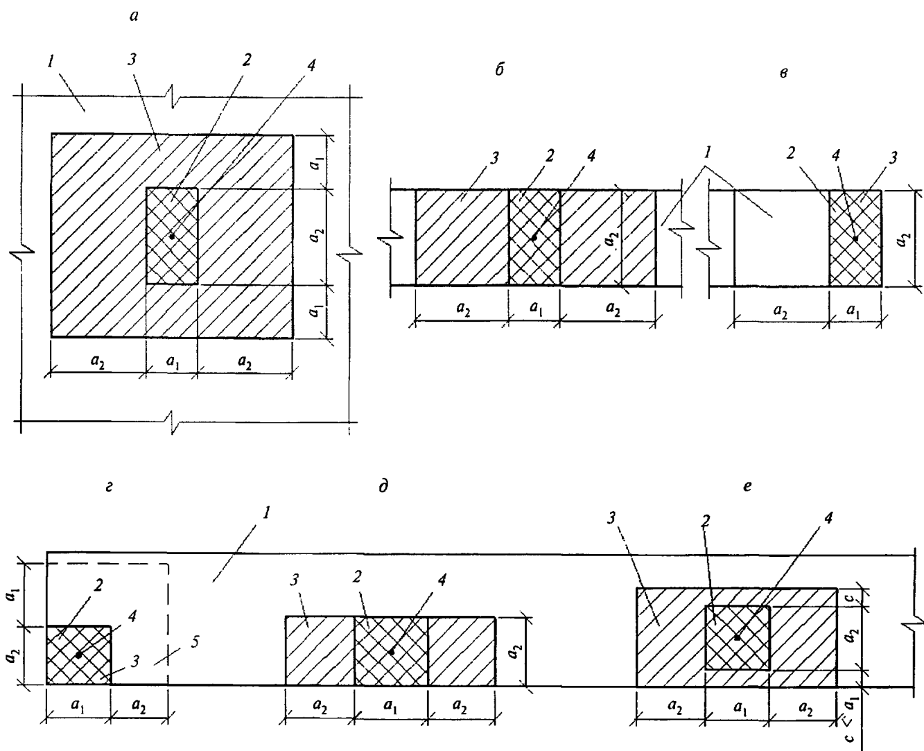
а — вдали от краев элемента; б — по всей ширине элемента; в — у края (торца) элемента по всей его ширине; г — на углу элемента; д — у одного края элемента; е — вблизи одного края элемента
