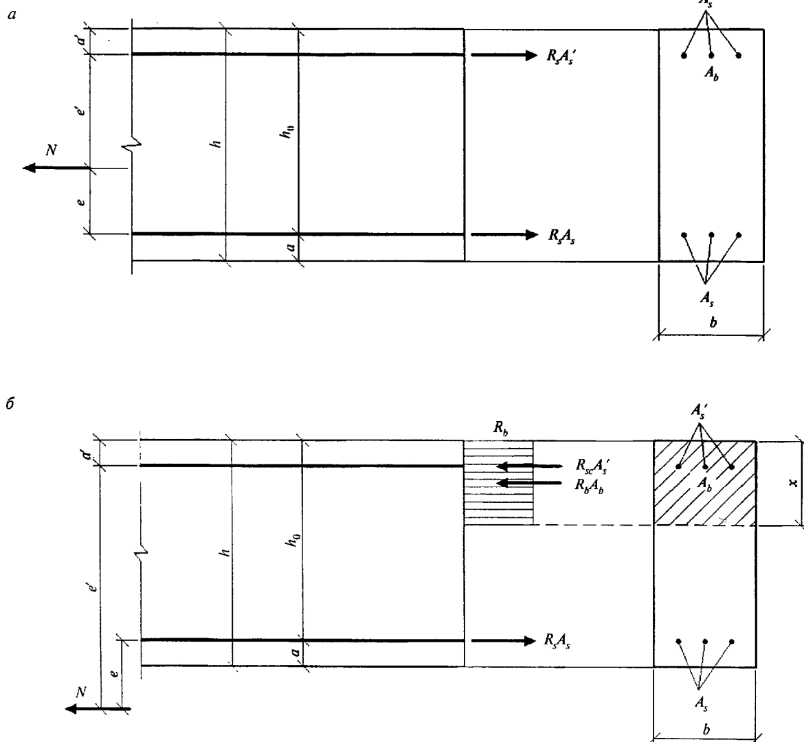
а — между равнодействующими усилий в арматуре S и S' ; б — за пределами расстояния между равнодействующими усилий в арматуре S и S'
