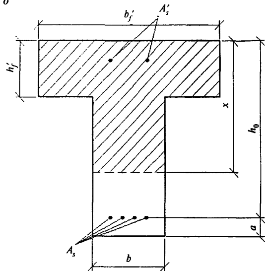
Рисунок 6.4 — Положение границы сжатой зоны в сечении изгибаемого железобетонного элемента
