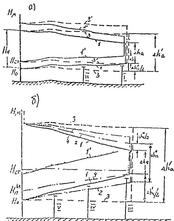
Рис. 2. Примерные асимметрические графики тепловой сети с автоматизированными ИТП:
