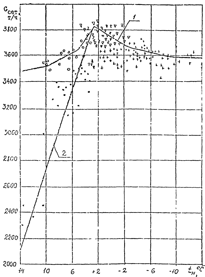
Рис. 1. Графики расхода сетевой воды в системе районного теплоснабжения при автоматизации отопления в ТП (1; • - весна) и без автоматизации (2; о - весна; +, ∇ - зима)
