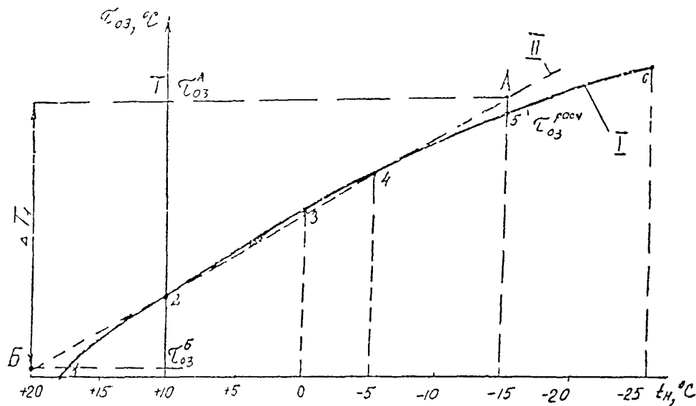
Рис. I. Графики для определения параметров настройки регулятора отопления "Электроника Р-ИМ" на заданный режим регулирования:
