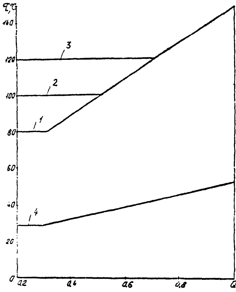
Рис. 5. Режим работы тепловой сети от котельной при автоматизации ГПП: 1 - обычно принимаемый график; 2, 3 - возможные графики; 4 - график обратной связи
