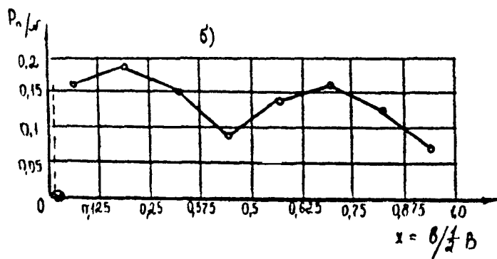
Рис. 8. Полигоны распределения вероятности возникновения повреждений кровли домов сер. I-515 на участках: а - по длине здания; б - по ширине здания; \odot - расположение воронок водосточа
