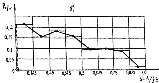
Рис. 5. Гистограммы распределения вероятности возникновения повреждений кровли домов сер 11-18 на участках: а - по длине здания; б - по ширине здан: л; ⊗ - расположение воронок водостока
