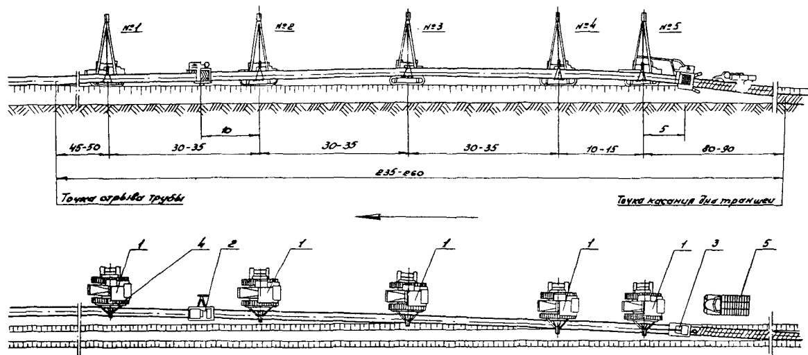
Рис. I. Расстановка машин в колонне при совмещенном способе изоляционно-укладочных работ:
