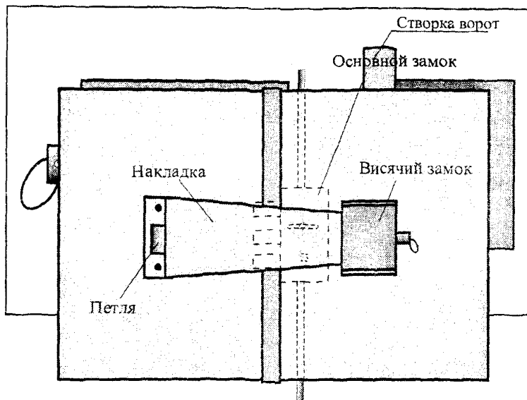
Рисунок 17 - Блокировка гаражных ворот
