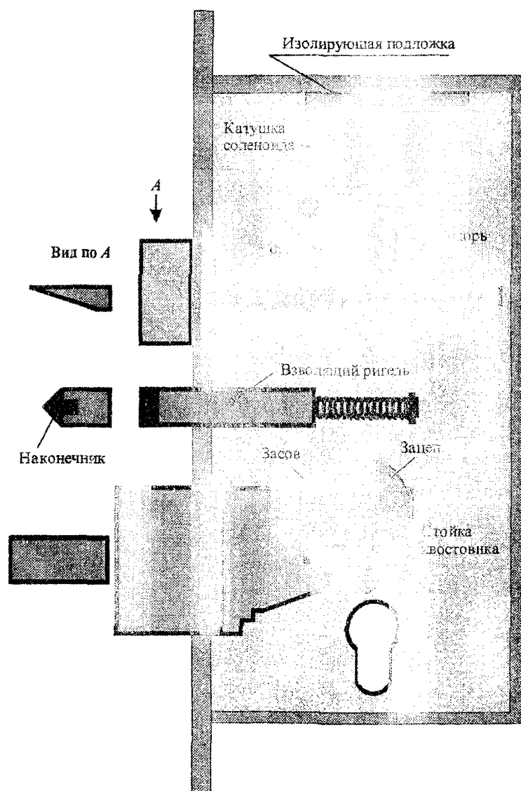
Рисунок 13 - Замок с электроблокировкой (рычаги и тяги не показаны)
