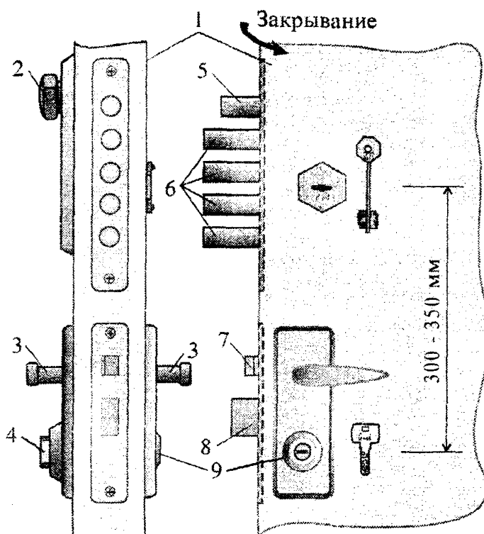
Рисунок 16 – Пример оборудования двери двумя врезными замками
