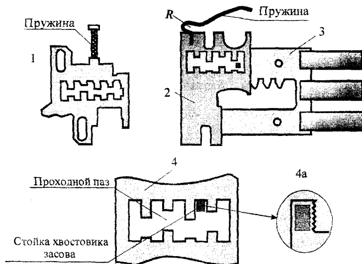
Рисунок 9 - Элементы сувальдных МС:
