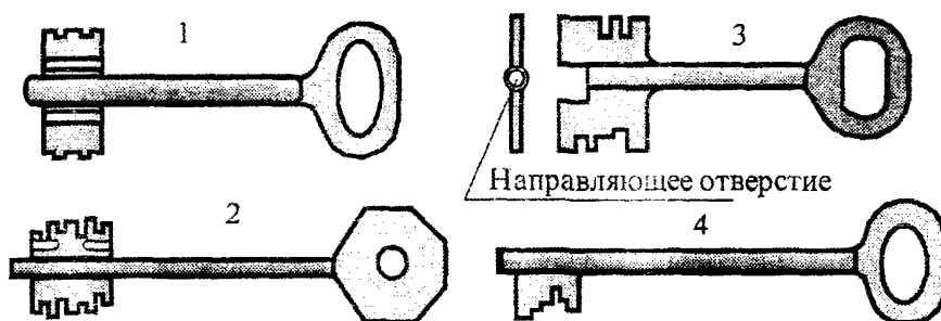
Рисунок 10 - Примеры ключей для сувальдных МС:
