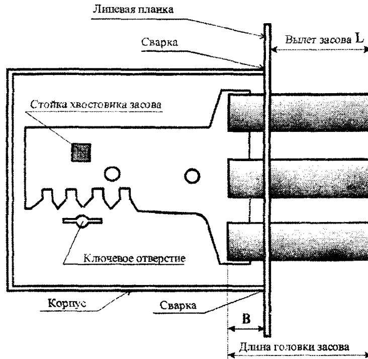
Рисунок 2 - Корпус врезного замка с размещенным в нем засовом
