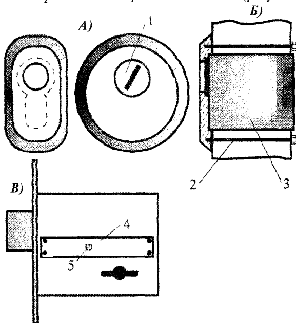
Рисунок 8 - Примеры защитных накладок от высверливания и сворачивания
