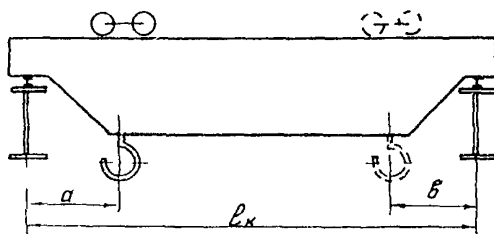
Рис.8. Схема расположения тележки
