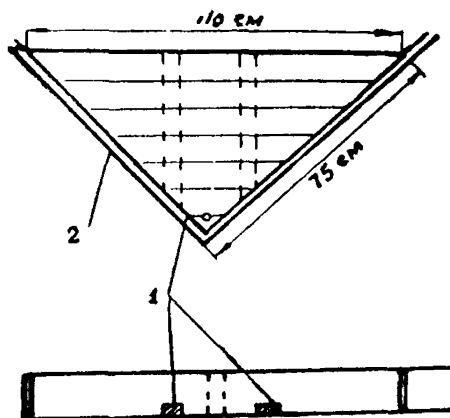
Рис 3 Деревянные щитовые буйки 1—поперечные рейки; 2—брус
