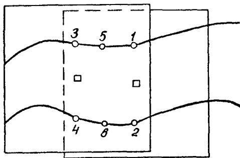
Рис. 8. Схема расположения точек при ориентировании снимков в стереометре
