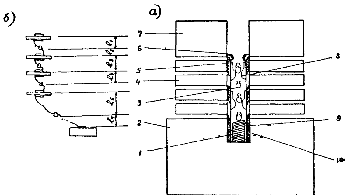
Рис. 1. Привязной буюк а—разрез буюка в собранном виде; б—развернутая схема привязного буюка 1—привязная леска; 2—бетонный корпус, 3—катушка; 4—шайба, 5—штулка, 6—пружина верхней шайбы, 7—верхняя шайба, 8—пружины, 9—катушка, 10—штулка
