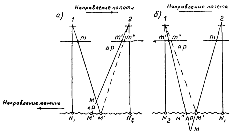
Рис. 2. Схема стереофотограмметрического измерения скорости течения*
