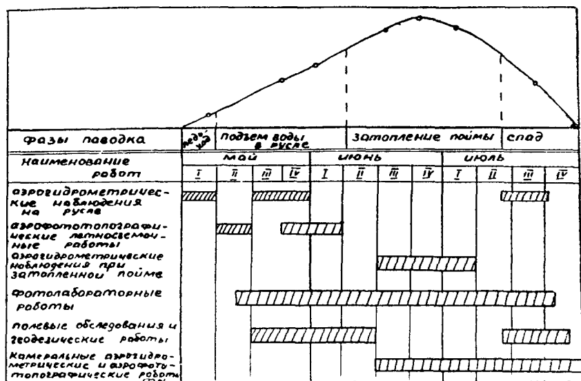
Рис. 14 Технологическая схема аэрогидрометрических работ
