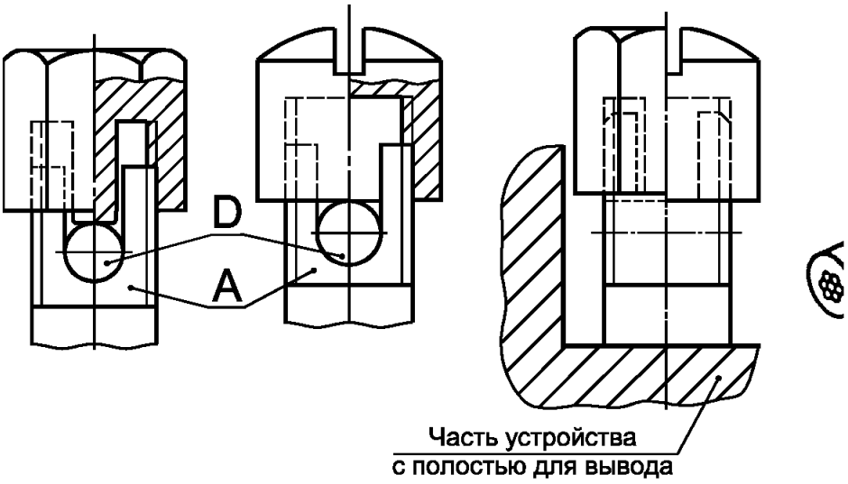
A — неподвижная часть; D — место для проводника
