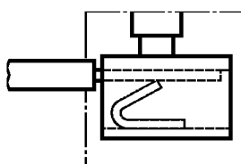
Рисунок D.7 — Безрезьбовые выводы
