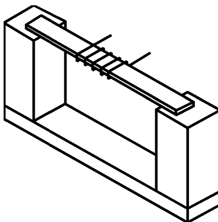
Рисунок М.1 — Приспособление для испытания нагретой проволокой
