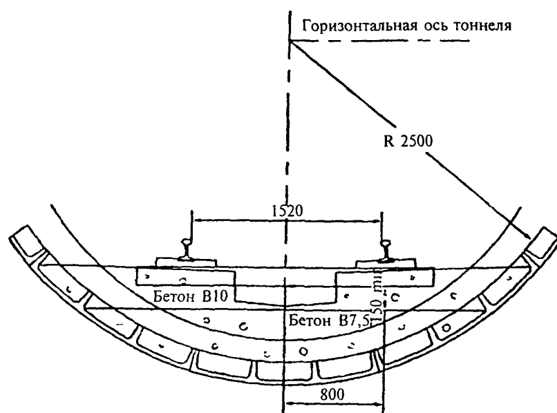
Перегонный тоннель с чугунной обделкой
