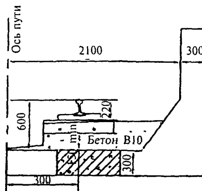
Станция мелкого заложения
