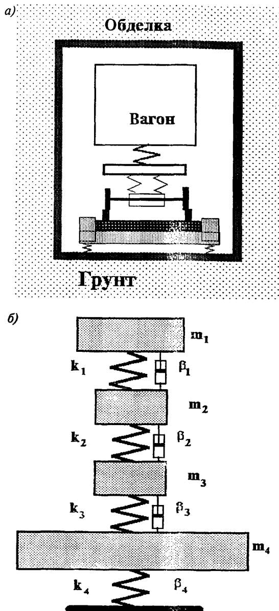
а — механическая схема; б — физическая модель системы
