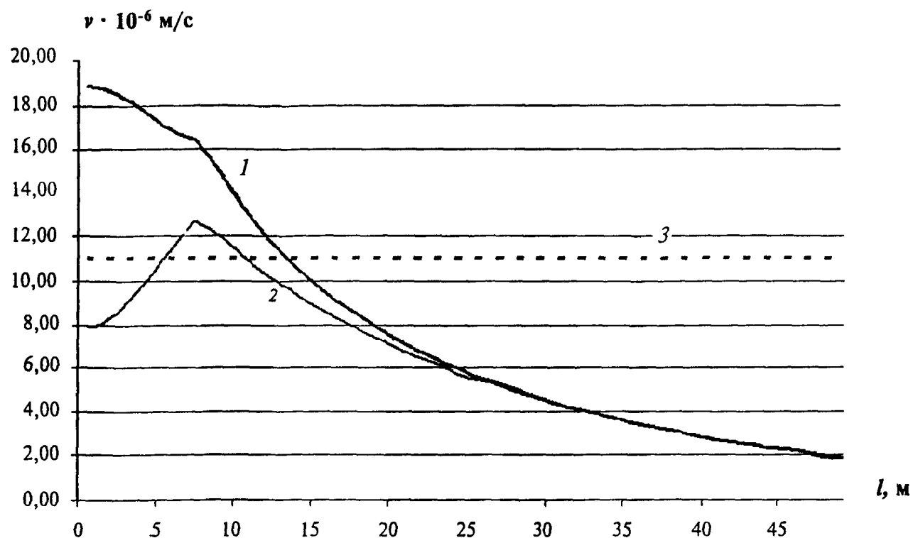
Рисунок Б.1 — Зависимость максимальной величины вертикальной и горизонтальной составляющих виброскорости v от расстояния до тоннеля l в октавном диапазоне 16 Гц
