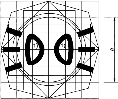
Рисунок 4.16а — Подфарник
