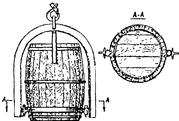
Захват для деревянных бочек
