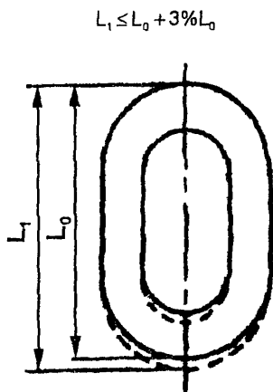
Рис. 1. Увеличение звена цепи: L_0 – первоначальная длина звена, мм; L_1 – увеличенная длина звена, мм
