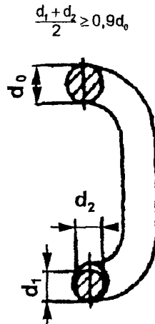
Рис. 2. Уменьшение диаметра сечения звена цепи: d_0 – первоначальный диаметр, мм, d_1, d_2 – фактические диаметры сечения звена, измеренные по взаимно перпендикулярным направлениям, мм
