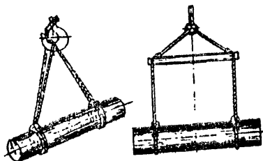
Полуавтоматическая строп-удавка
