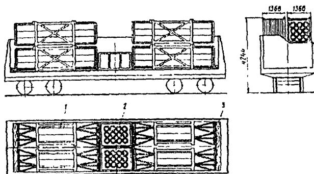
Рис 33 1 – контейнер СТ7-5М для труб, 2 – контейнер СТ6-3 для муфт 3 – упорный брус
