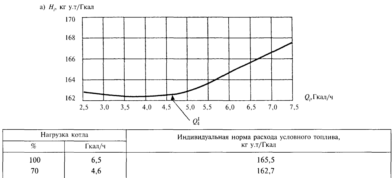
Рисунок 1 — Нормативная характеристика котла ТВГМ-30 (топливо — природный газ)
