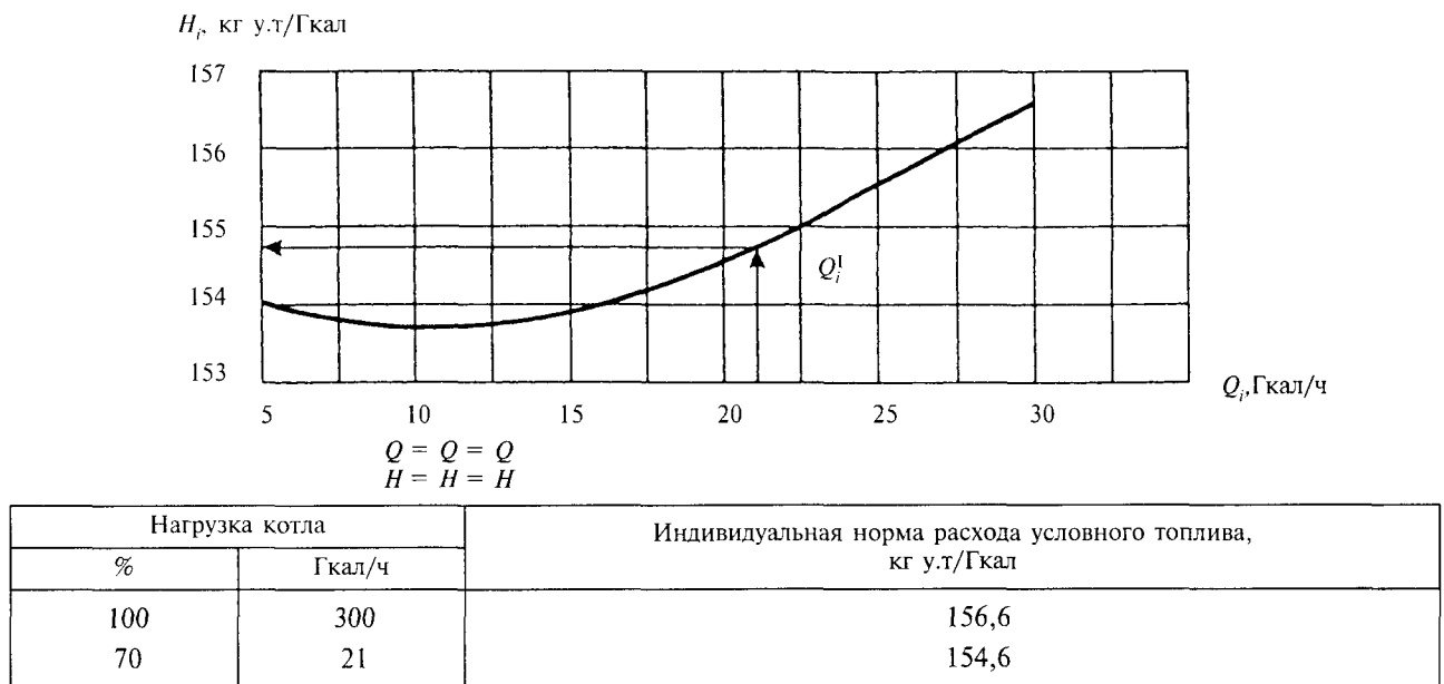
Рисунок 1 — Нормативная характеристика котла ТВГМ-30 (топливо — природный газ)
