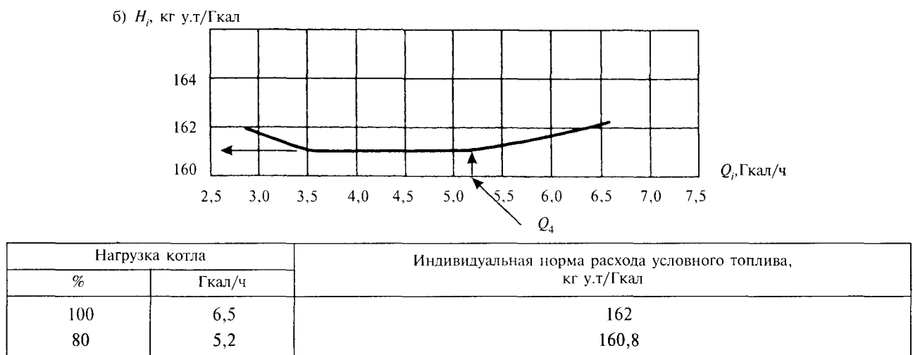
Рисунок 2 — Нормативная характеристика котла ДКВР-10-13
