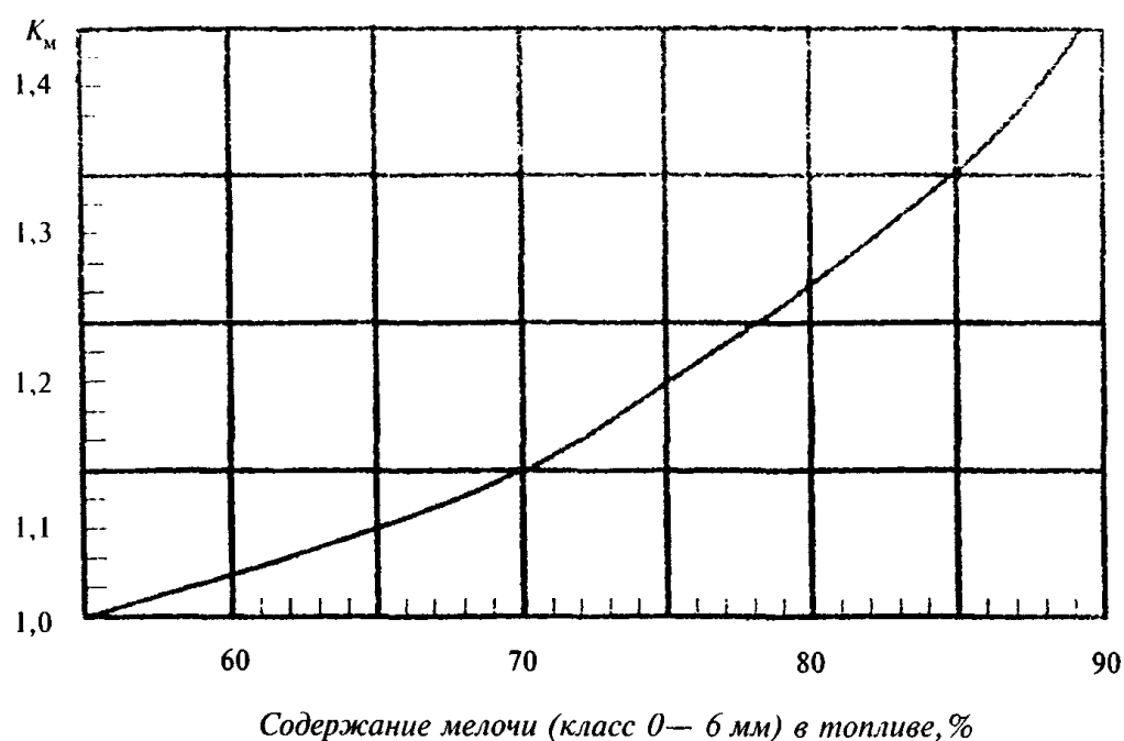
Рисунок 2 — Поправки на содержание мелочи в топливе ( K_m )
