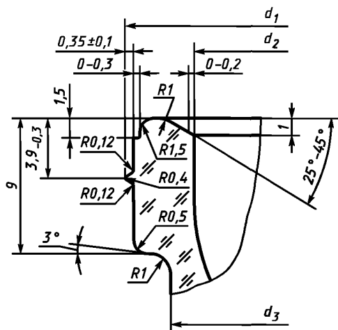
Рисунок 2 — Венчик типа I
