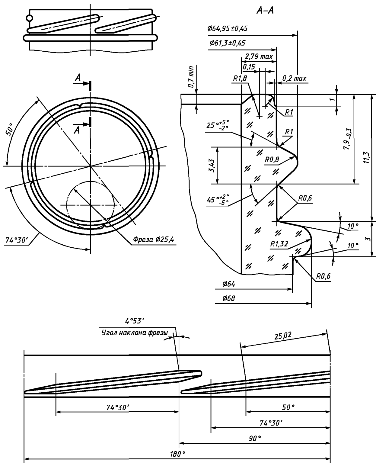
Рисунок 4 — Венчик типа III-1
