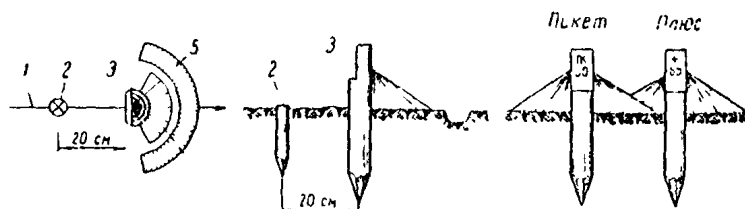
Рис 9 Закрепление пикетажа
