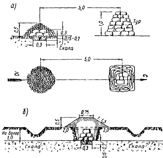
Рис. 16. Марка, закладываемая в скалу горизонтального залегания:
