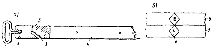
Рис 1. Измерительная лента а — оформление конца ленты, б — нумерация лицевой и оборотной сторон ленты
