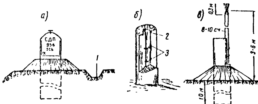
Рис. 12. Схемы знаков, закрепляющих трассу: а — осевой столб; б — столб с железными скобами для постановки маячной вехи; в — маячная веха 1 — канавка по кругу; 2 — желоб для постановки жерди; 3 — скобы
