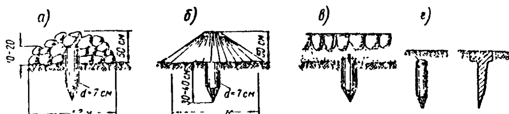
Рис. 13. Закрепление трассы в безлесной или обжитой местности: а — каменная наброска; б — земляной конус с потайной точкой; в — на существующей мощеной дороге (деревянным колом); г — на грунтовой дороге (деревянным колом или ж.-д. костылем)
