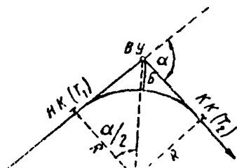
Рис. 19. Схема элементов закругления
