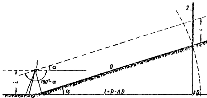
Рис. 5. Схема измерения углов наклона эклиметром: 1 — эклиметр; 2 — вешка по отвесу
