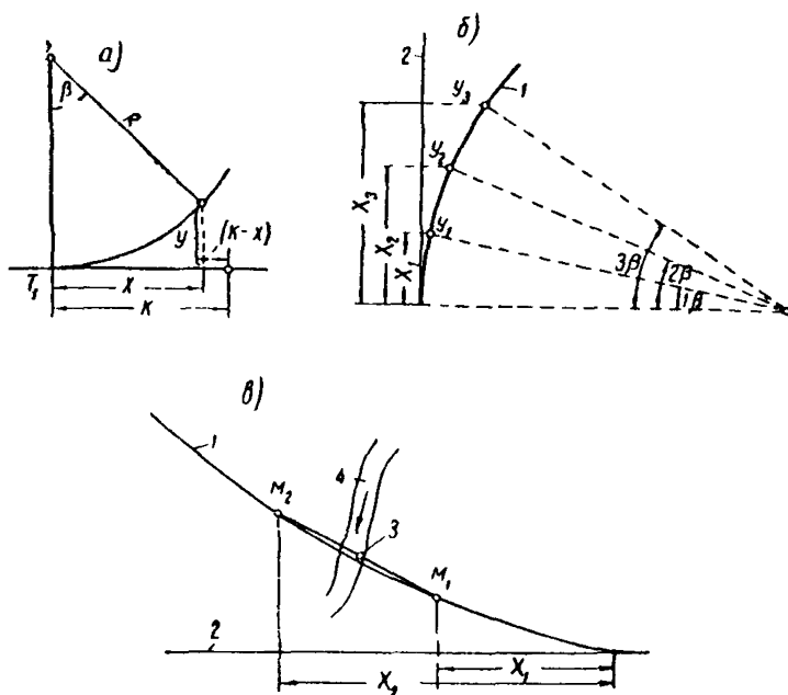
Рис. 22. Схема выноски точек на кривую: а и б — выноски пикетных точек с касательной на кривую методом ординат; в — фиксирование характерных точек на кривой:
