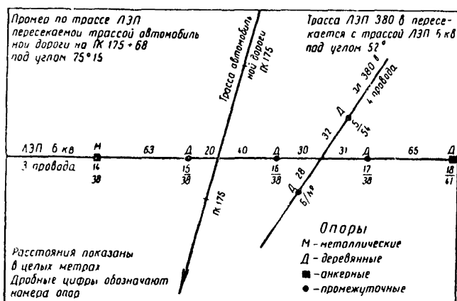
Рис. 25. Промер по трассе ЛЭП (образец заполнения журнала)
