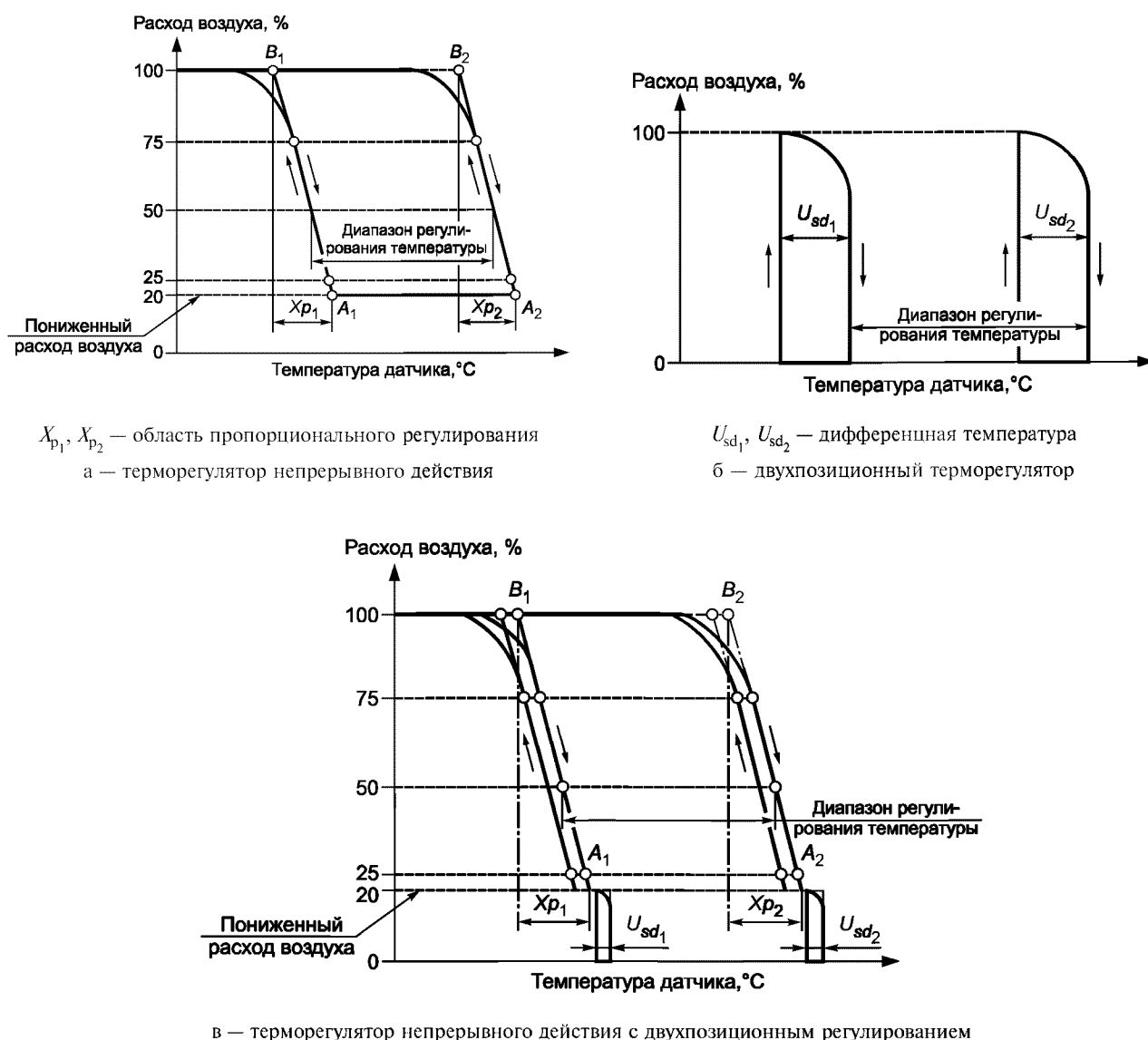
Рисунок 2 — Типовые характеристики терморегуляторов
