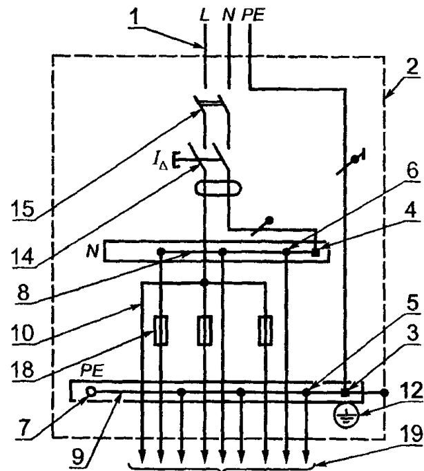
Рисунок А 4 — Схема квартирного группового щитка (для хозблока), присоединенного к квартирному учетно-групповому щитку жилого дома
