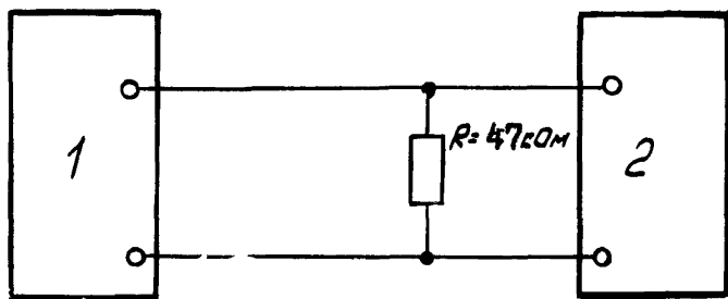
1 — электрогитара, 2 — милливольтметр, R — нагрузочное сопротивление
