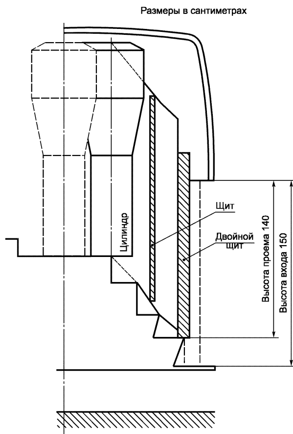
Рисунок 17 — Служебная дверь (см. 5.7.1.4)
