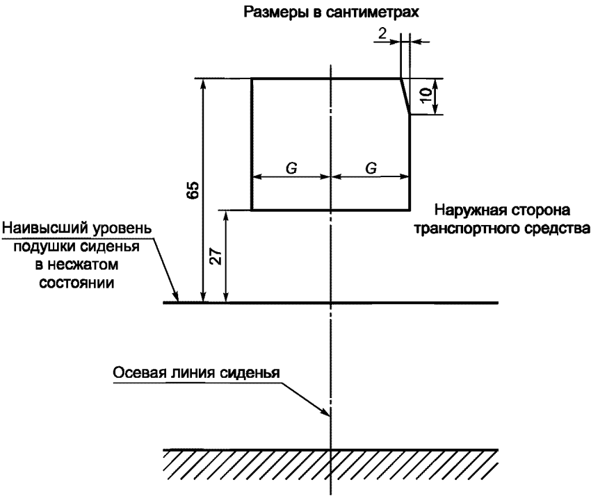
Рисунок 12 — Размеры сидений для пассажиров (см. 5.7.8.2)
