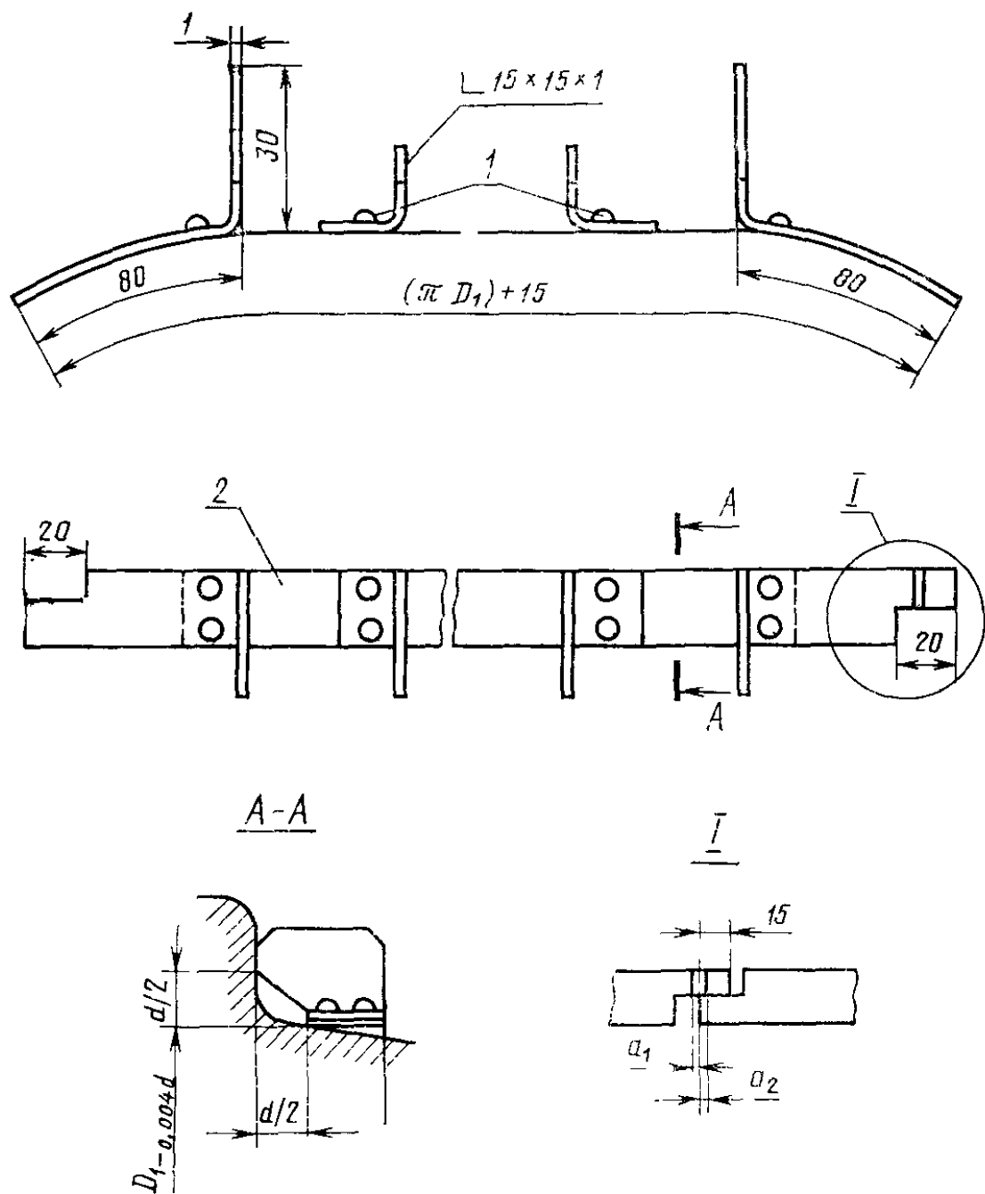
1—заклепка с потайной головкой; 2—лента 15×0,5
