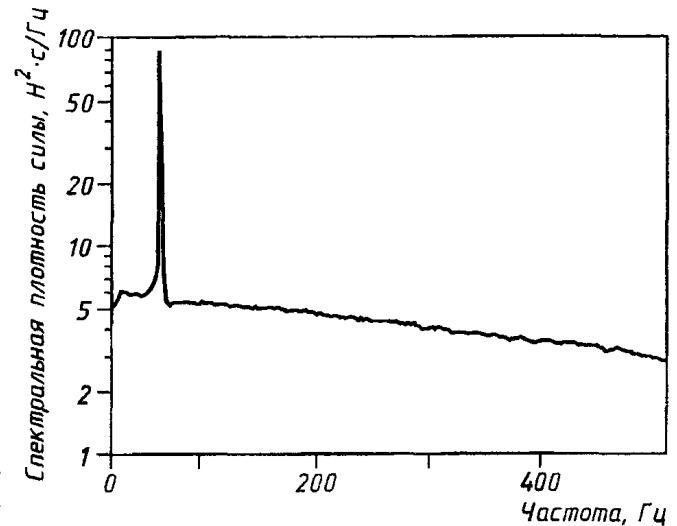
б) Спектральная плотность энергии сигнала силы с шумом
