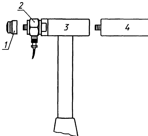
1 — сменная насадка; 2 — датчик силы; 3 — основная масса; 4 — сменная масса
