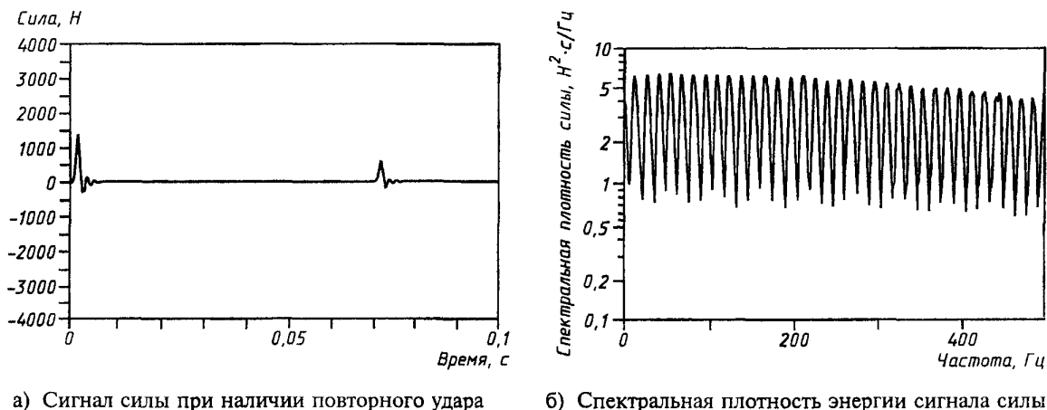
Рисунок 5 — Влияние повторного удара на спектр силы
