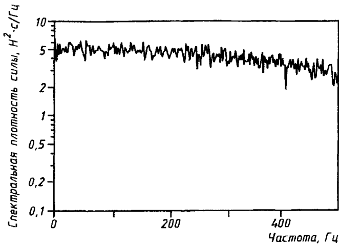
а) Спектральная плотность энергии в отсутствие окна силы
