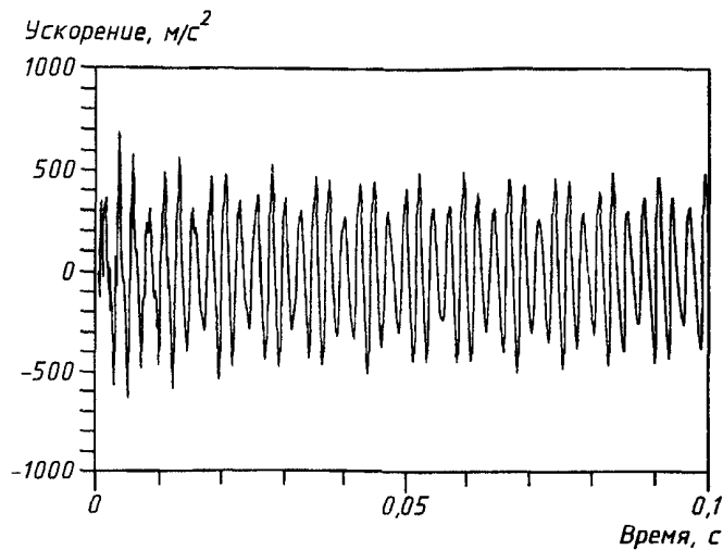
а) Сигнал ускорения
