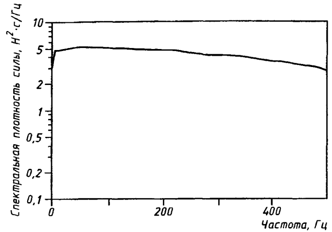
б) Спектральная плотность энергии при использовании окна силы
