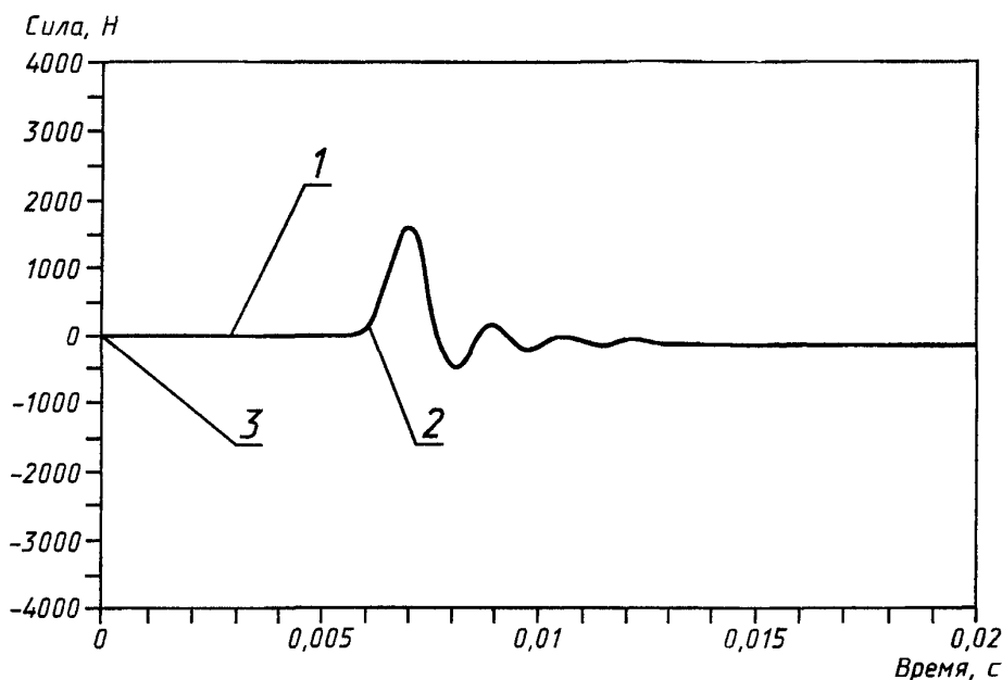
Рисунок 6 — Запись сигнала силы с нулевым участком вначале
