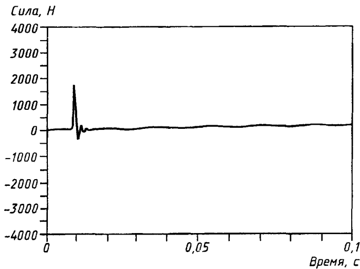
а) Сигнал силы в присутствии периодического шума
