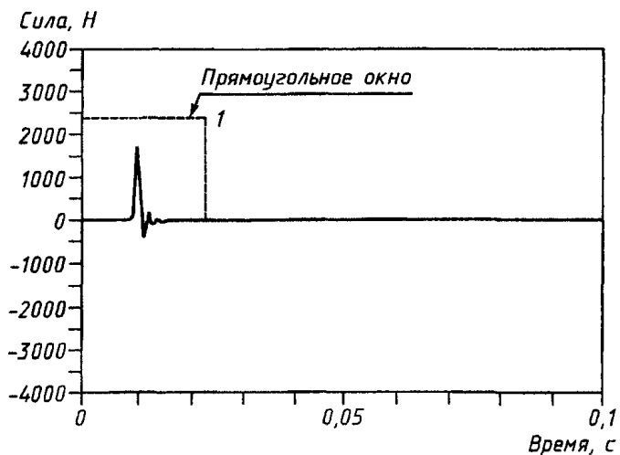
в) Сигнал силы после применения окна силы
