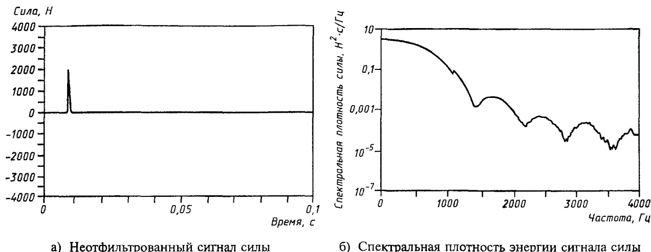
Рисунок 3 — Типичный импульс силы и его спектр
