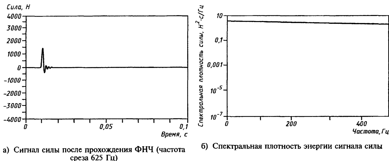
Рисунок 4 — Влияние низкочастотной фильтрации на сигнал силы и его спектр
