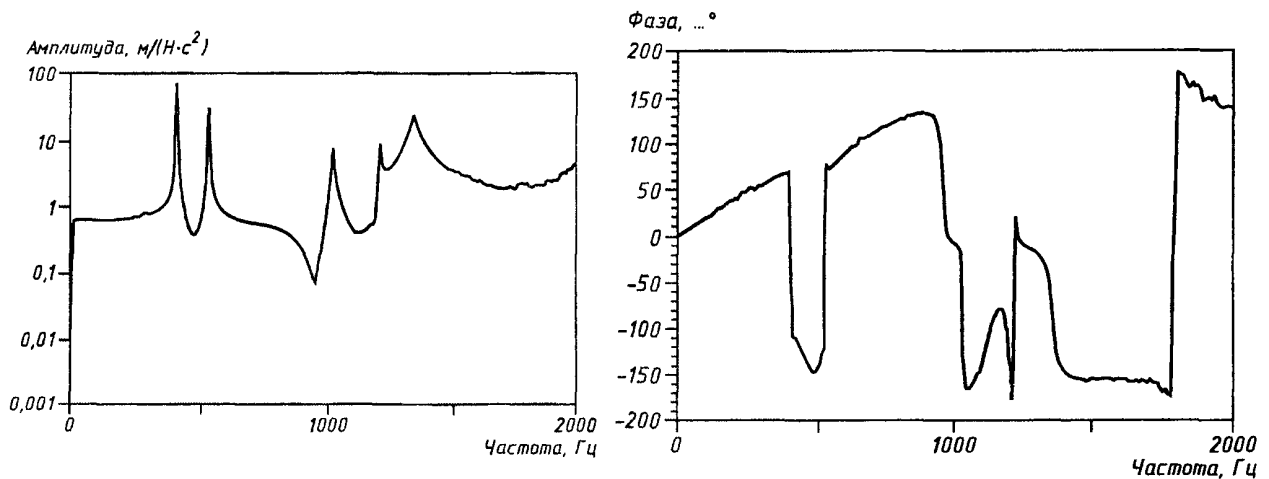
б) Ускоряемость (амплитуда и фаза) в отсутствие окна
