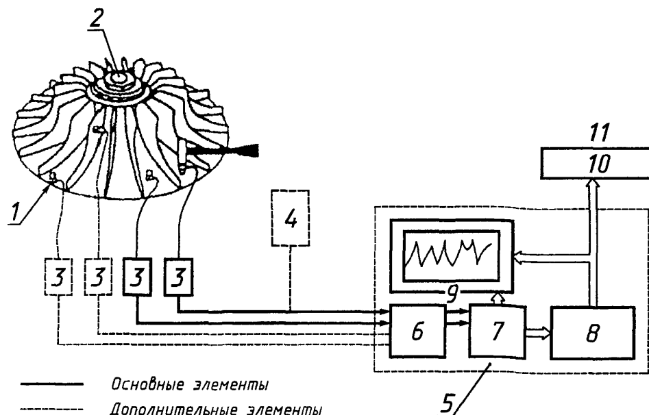
1 — датчик вибрации; 2 — испытуемая конструкция; 3 — устройства согласования; 4 — запоминающий осциллограф; 5 — блок анализа; 6 — ФНЧ; 7 — АЦП; 8 — ДПФ, расчет частотной характеристики устройства; 9 — дисплей; 10 — печатающее устройство; 11 — выходное устройство
