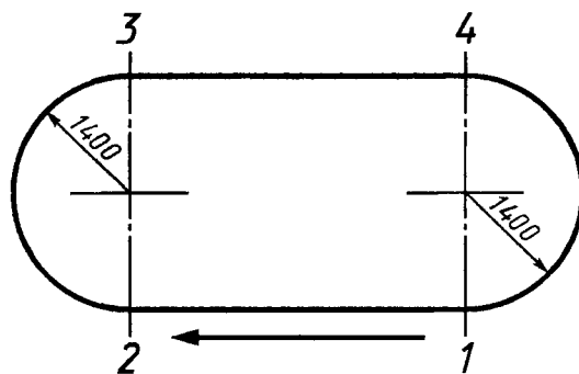
Рисунок А.1 — Испытательный полигон
