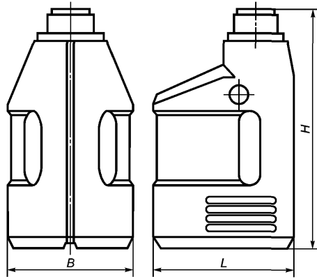
Бутылка БТ Ш-1-27 Рисунок А.27
