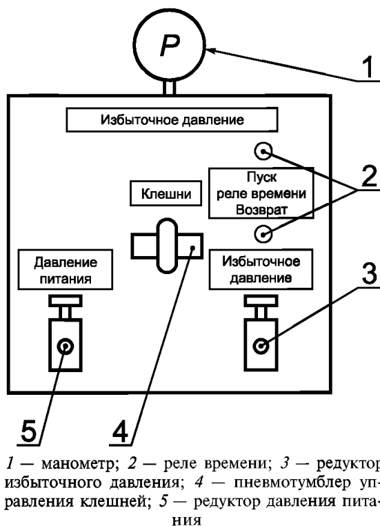
Рисунок М.2 — Схема пульта управления станком для испытания тары на герметичность под давлением
