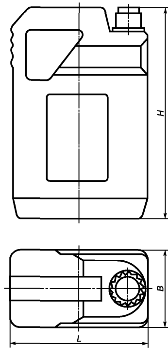
Канистра КН I-1-29 Рисунок А.29
