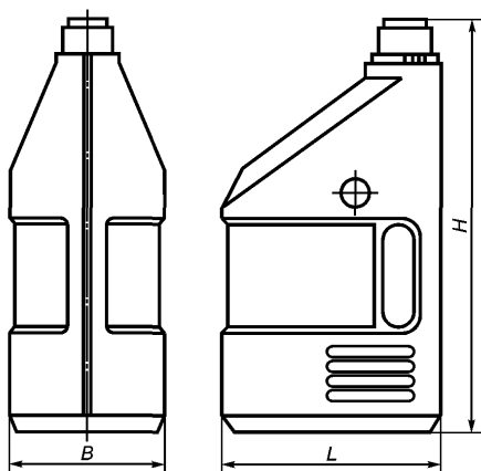
Канистра КН II-1-32 Рисунок А.32
