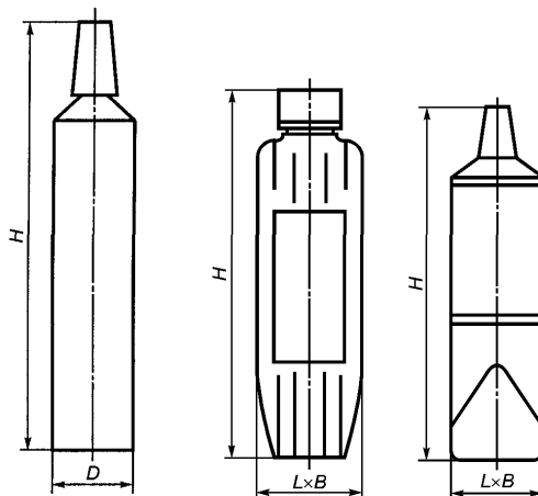
Туба ТБ I-1-33 Рисунок А.33
