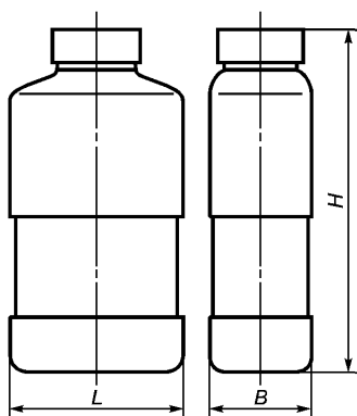
Банка БН II-1-7 Рисунок А.7
