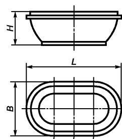
Банка БН IV-2-17 Рисунок А.17
