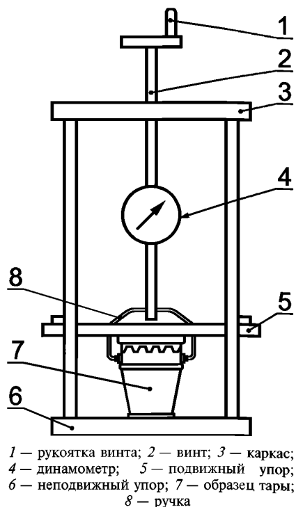
Рисунок 7 — Принципиальная схема универсального устройства для испытания прочности ручки и крепления ручки
