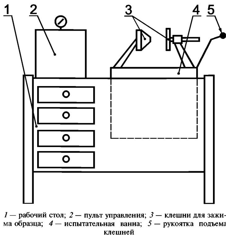
Рисунок М.1 — Схема конструкции станда для испытания тары на герметичность под давлением
