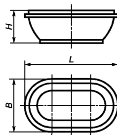
Банка БН IV-2-17 Рисунок А.17
