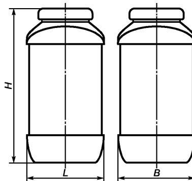
Банка БН II-2-8 Рисунок А.8
