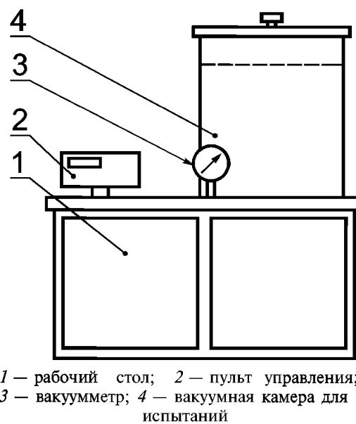
Рисунок М.3 — Схема внешнего вида станка для испытаний тары на герметичность под вакуумметрическим давлением
