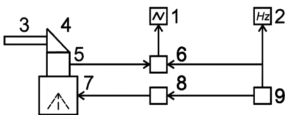
1 — индикатор (осциллограф); 2 — частотомер; 3 — испытываемое изделие; 4 — согласующий держатель; 5 — пьезоэлектрический детектор резонансных частот; 6, 8 — усилитель; 7 — вибратор; 9 — генератор звуковых частот
