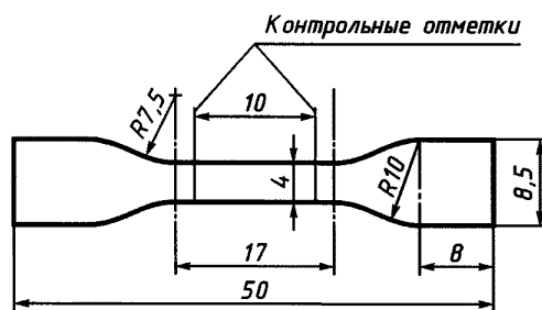
Рисунок 13 — Образец в виде двусторонней лопатки уменьшенного размера
