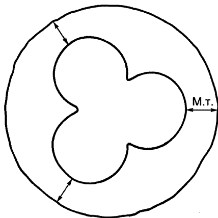
Рисунок 8 — Измерение оболочки (внутренний профиль некруглой формы)
