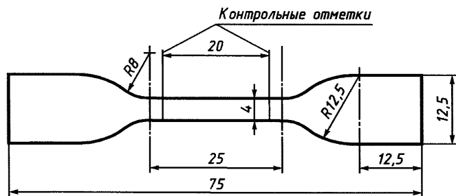
Рисунок 12 — Образец в виде двусторонней лопатки
