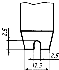
Рисунок 14 — Конец вырубного ножа с выемкой
