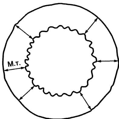
Рисунок 3 — Измерение толщины изоляции (многопроволочная жила)
