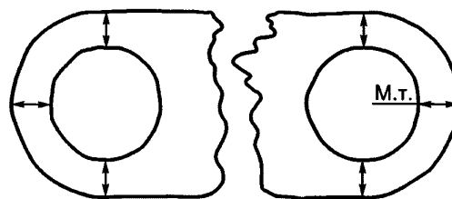
Рисунок 11 — Измерение толщины оболочки (плоский кабель с разделенными жилами)
