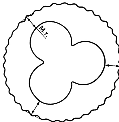
Рисунок 9 — Измерение толщины оболочки (наружная поверхность неправильной формы)
