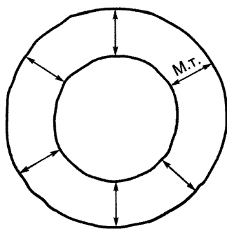
Рисунок 1 — Измерение толщины изоляции или оболочки (круглый внутренний профиль)
