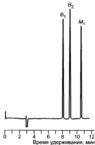
Рисунок 2 — Хроматограмма рабочего раствора смеси афлатоксинов
