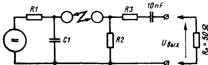
Принципиальная схема генератора 5/50 ns, U_{\text{вых}} = \pm 0,5 \text{ kV} до 4 kV, частота повторений 5 kHz (2,5 kHz при 4 kV)
