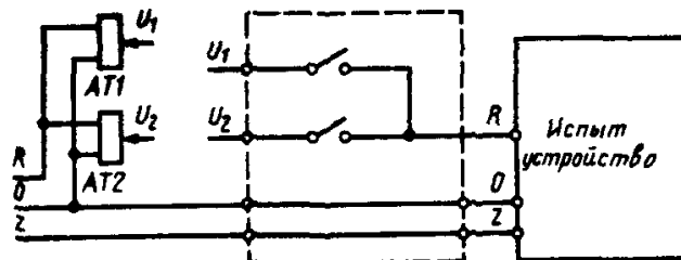
AT1, AT2—автотрансформаторы провал, когда U_1 = U_n U_2 < U_1 U_2/t_z , перенапряжение U_1 = U_n U_2 > U_1 U_2/t_z , отключение U_1 = U_n U_1 = 0/t_z t_z — продолжительность помехи
