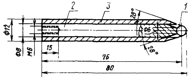
1—стальной шарик диаметром 8 мм; 2—латунный стержень; 3—изолятор
