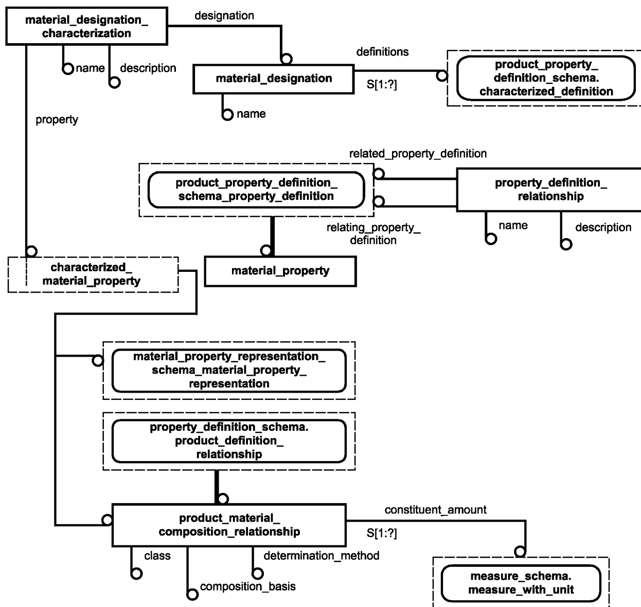
Рисунок D.1 — material_property_definition_schema — EXPRESS-G диаграмма 1 из 1
