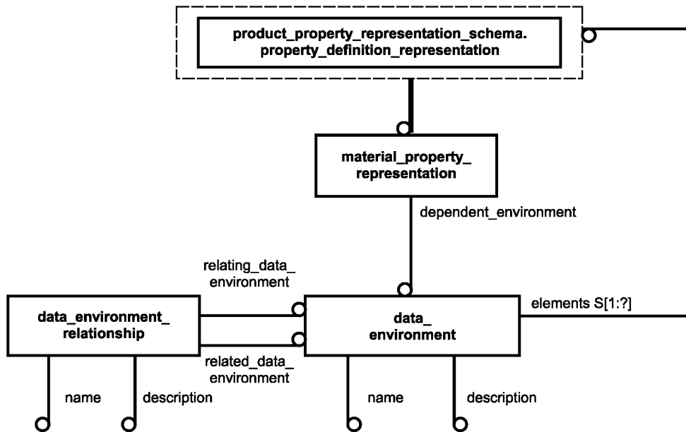
Рисунок D.2 — material_property_representation_schema — EXPRESS-G диаграмма 1 из 1
