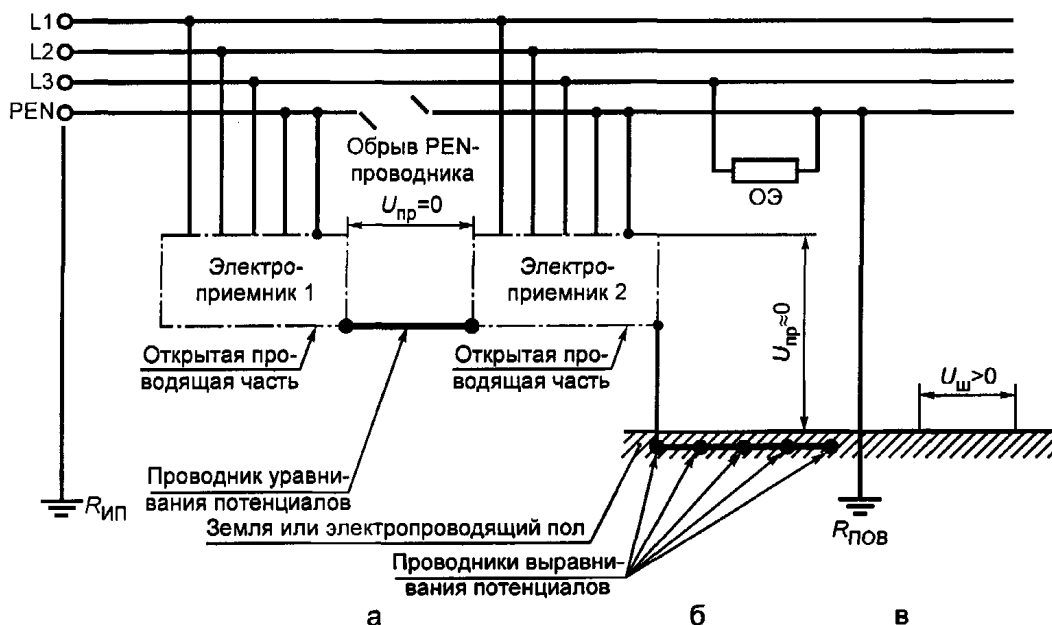
Рисунок В.2 — Сеть TN-C с оборванным PEN-проводником
