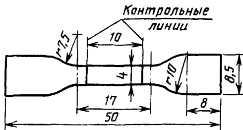
Образец в виде двусторонней лопатки уменьшенного размера
