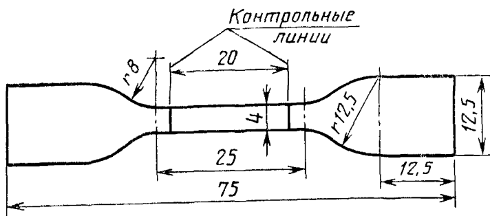
Образец в виде двусторонней лопатки
