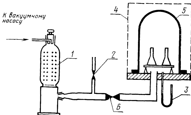
1—осушительная колонка, 2—вентиль соединяющий установку с атмосферой, 3—манометр, 4—предохранительная проволоочная сетка, 5—вакуумная камера, 6—затвор насосного трубопровода
