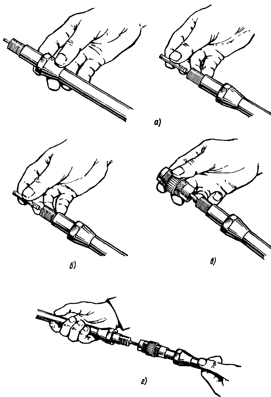
Рис. 6.10. Монтаж соединителя типа СКП
