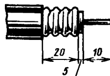
Рис. 6.12. Разделка кабелей
