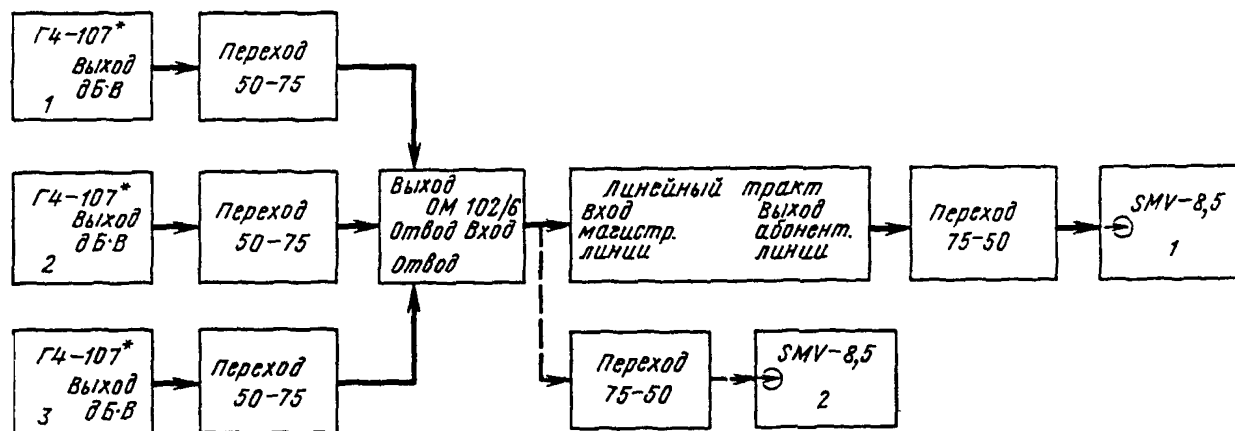
Рис. 7.7. Структурная схема измерения отношения сигнала к помехе комбинационной частоты третьего порядка \text{IMA}_{\text{III}}(n)
