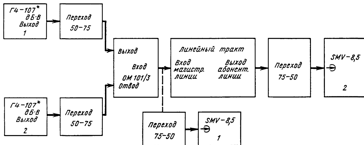
Рис. 7.10. Структурная схема измерения отношения сигнала к помехе комбинационной частоты второго порядка \text{ИМА}_{\text{II}(B)}
