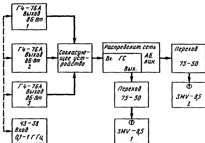
Рис. 7.5. Структурная схема измерения сигнала к помехе комбинационной частоты третьего порядка \text{IMA}_{\text{III}}(\kappa) в дециметровом диапазоне
