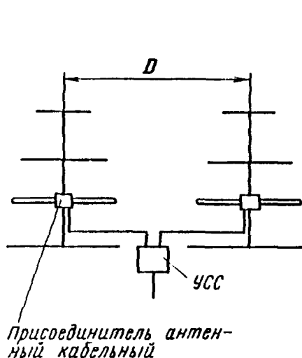
Рис. П.1.1. Сдвоенная антенна
