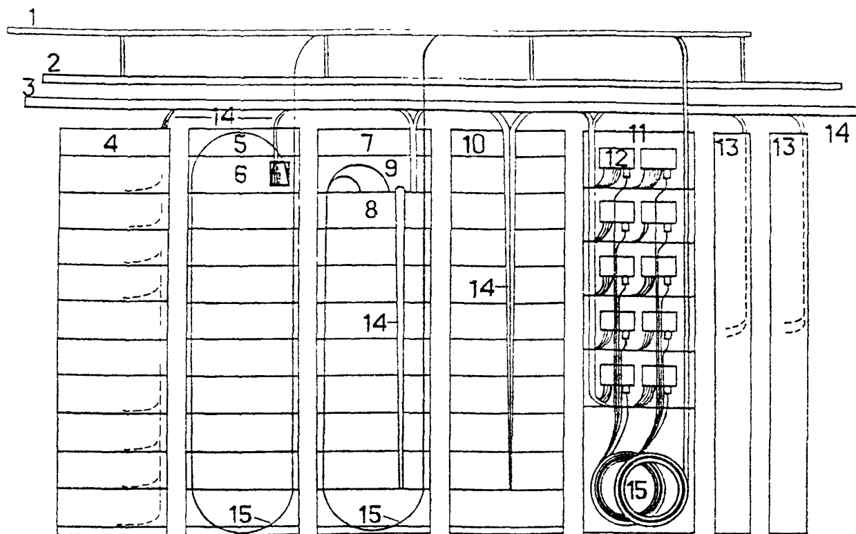
Рис. 14. Схема расположения оконечных устройств ВОЛС на стойках в типовом ЛАЦ (вид с тыльной стороны стоек):
