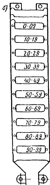
Рис. 17. Нумерация пар на кабельном боксе 100х2
