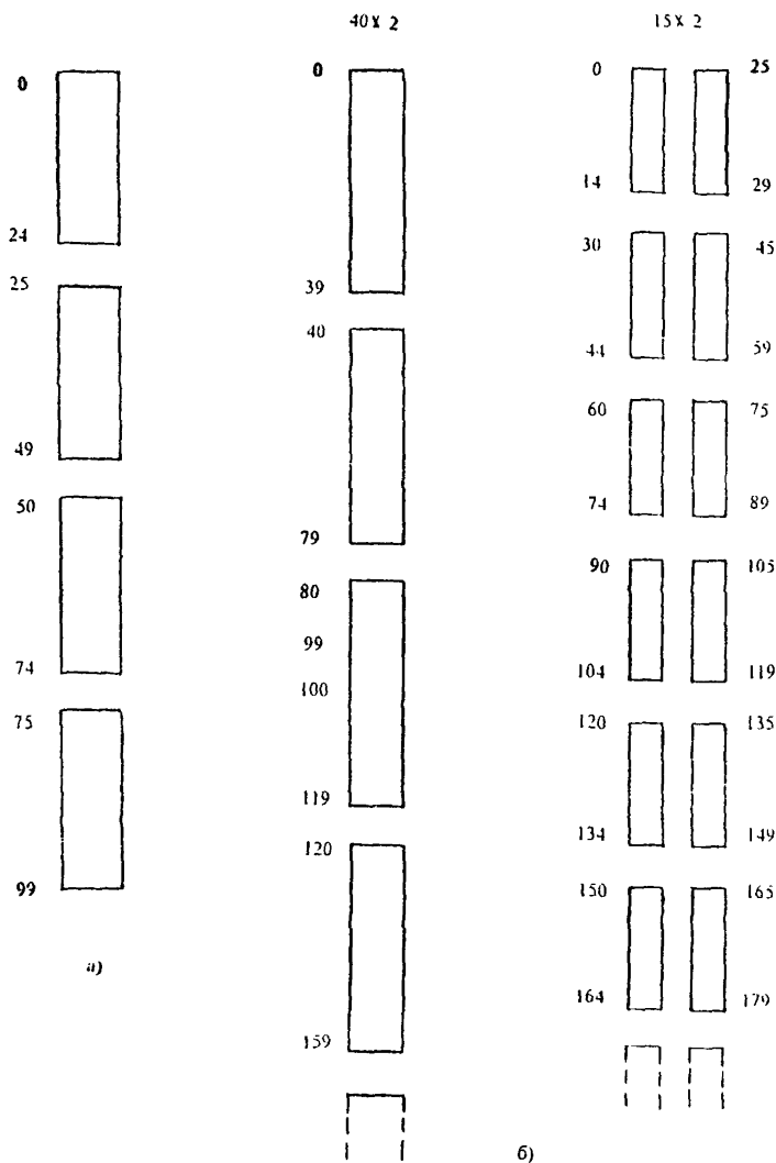
Рис. 16. Нумерация пар на оконечных кабельных устройствах кросса: а) защитных полосах 25х2 абонентского кросса; б) рамках 40х2 и 15х2 кросса соединительных линий
