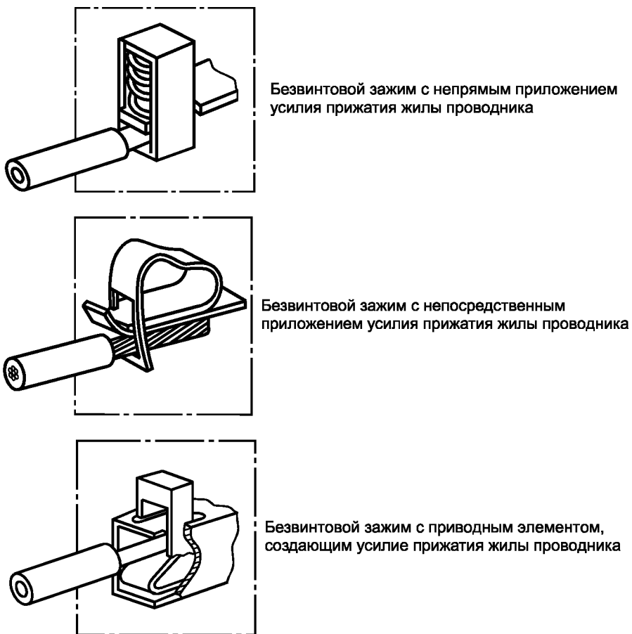
Рисунок 6 — Примеры безвинтовых контактных зажимов
