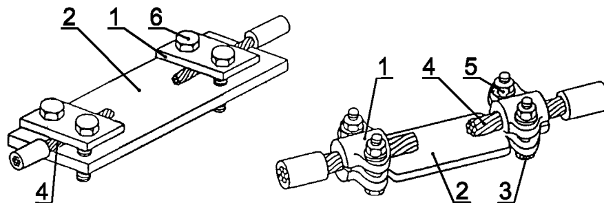
Рисунок 4 — Зажимы с прижимной пластиной
