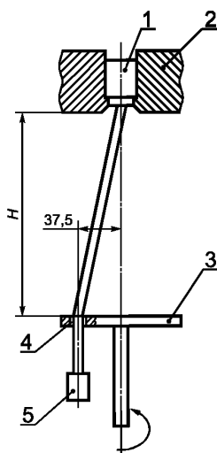
1 — зажим; 2 — подставка; 3 — плата; 4 — втулка; 5 — груз
