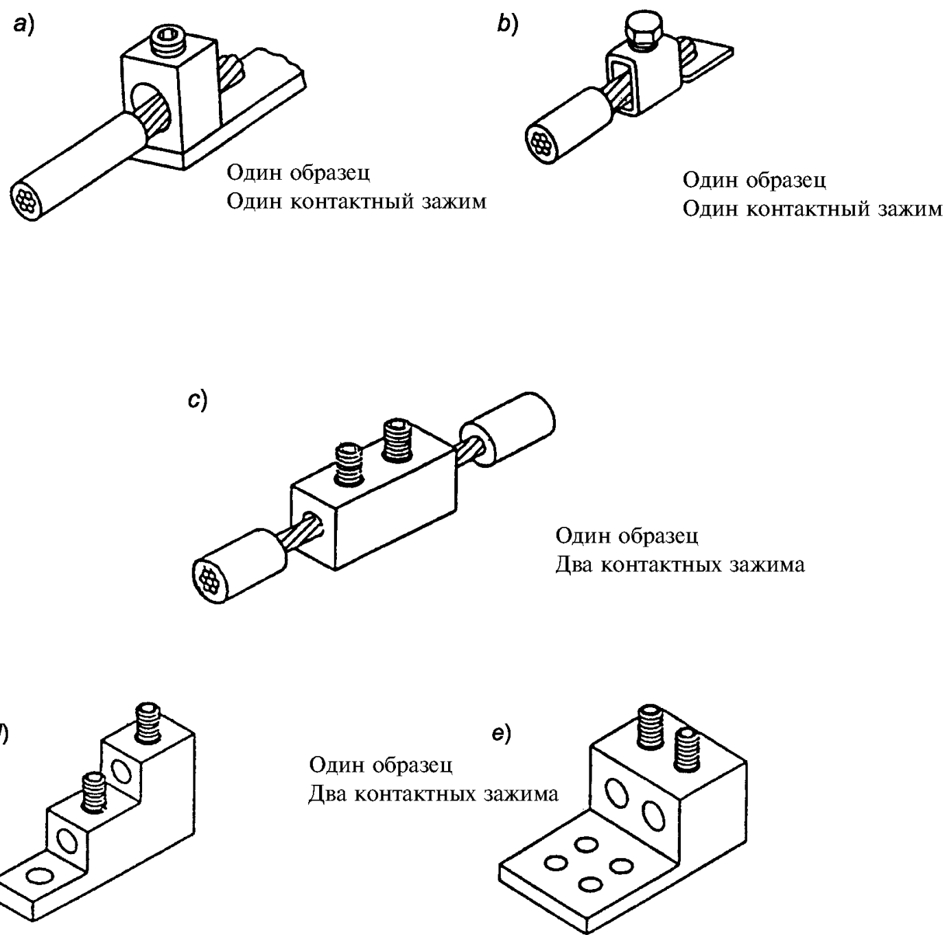
Рисунок F.3 — Торцевые зажимы с непосредственным зажимом проводника(ов)
