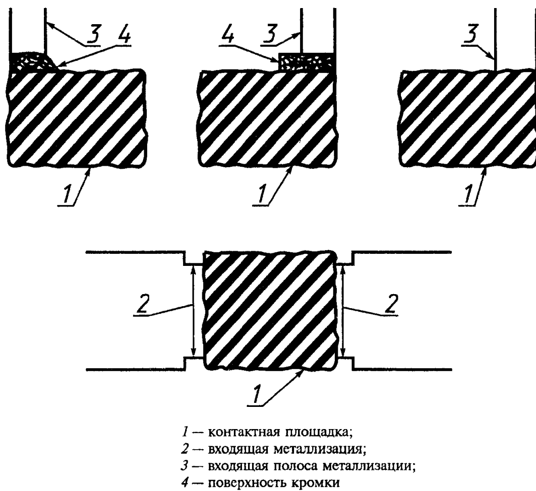
Рисунок 5 — Зоны контактных площадок
